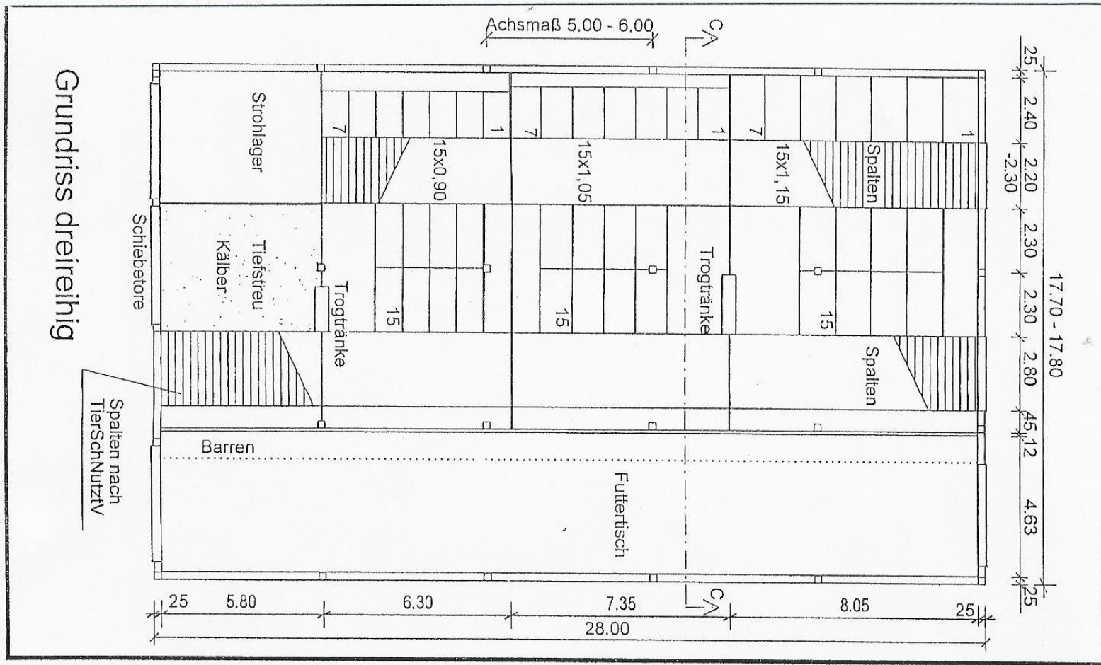
dreireihiger Liegeboxen- laufstall
