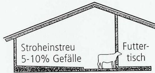
Tretmiststall
