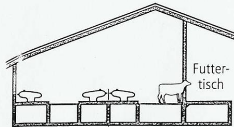
Boxenlaufstall dreireihig
